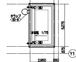
階段室屋根伏図 1:100
