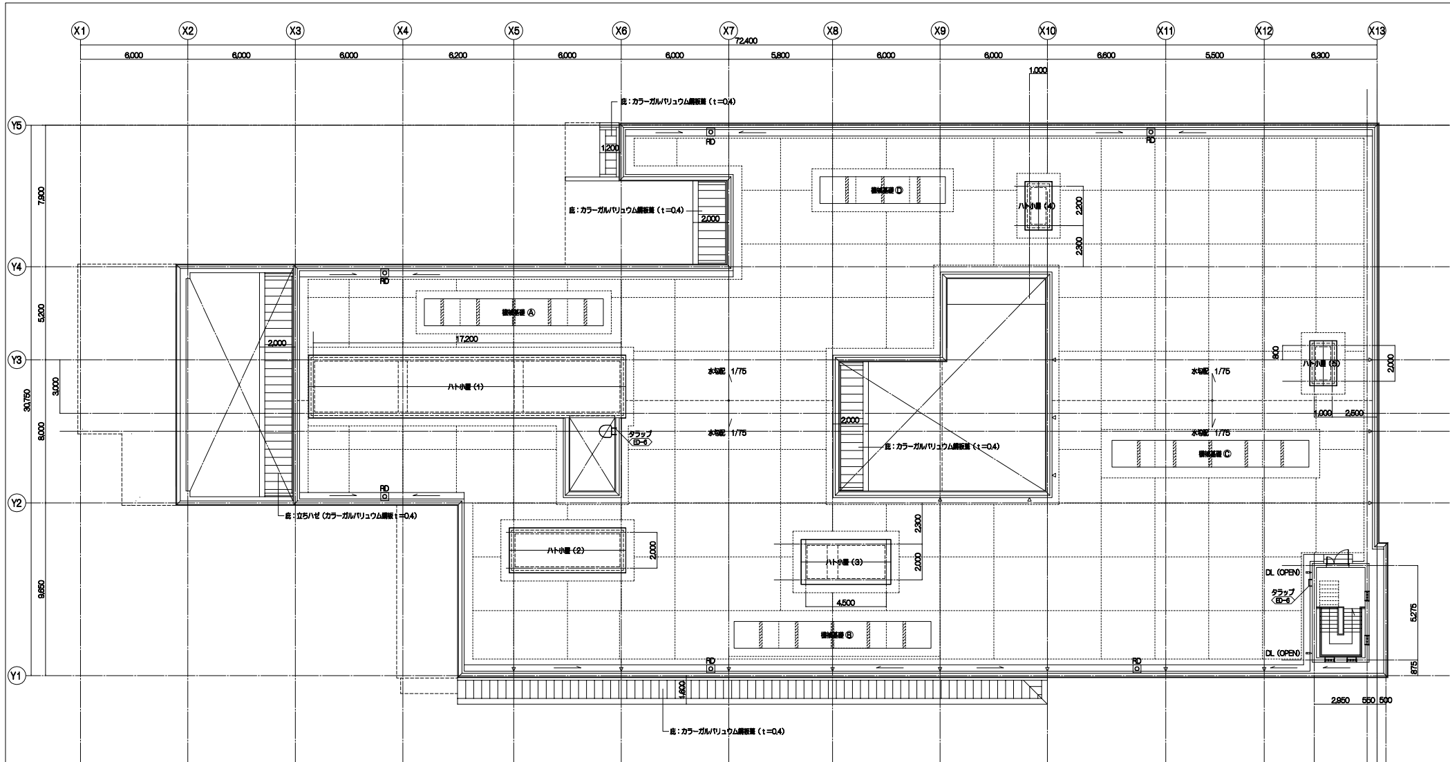
屋根伏図 1:100
